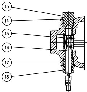
A-A Section
